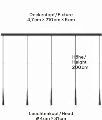
5 Pendel / 5 Pendants
