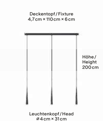
3 Pendel / 3 Pendants
