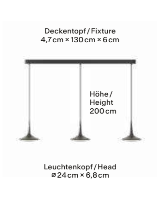
3 Pendel / 3 Pendants
