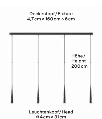
4 Pendel / 4 Pendants
