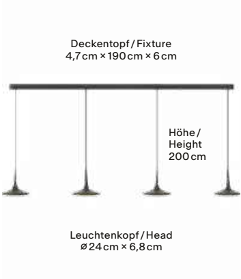
4 Pendel / 4 Pendants
